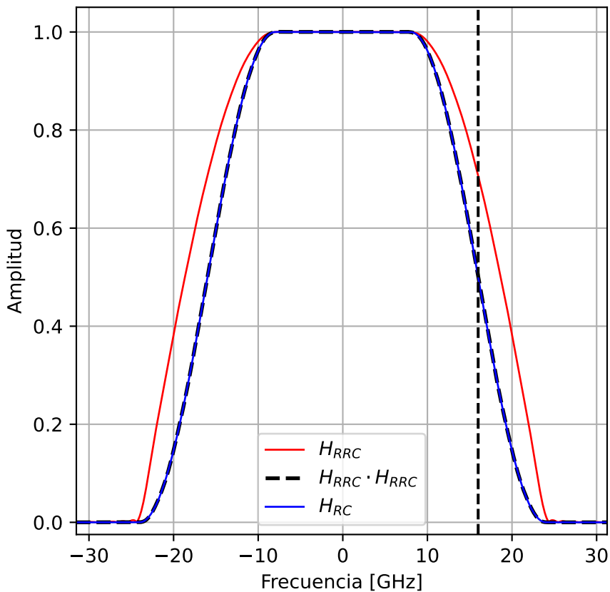
Respuesta en Frecuencia del RC y RRC. \beta = 0.5
